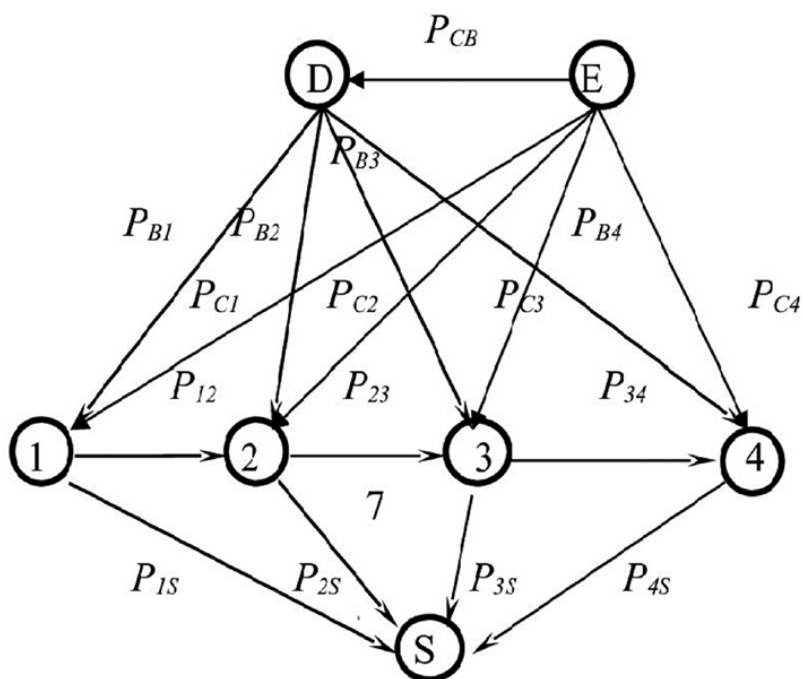
Рис. 1. Потокковая диаграмма для анализа надежности функционирования восстанавливаемого двигателя внутреннего сгорания: D — водитель; E — внешняя среда; 2 — система контроля; 3 — аппаратура топливоподачи; 4 — цилиндропоршневая группа; 5 — кривошипно-шатунный механизм; S — сток
